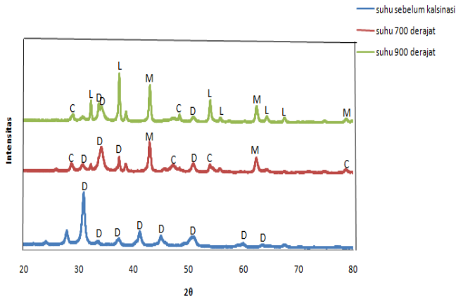
Gambar 1 Pola difraksi dolomit kalsinasi pada berbagai temperatur. D = CaMg(CO 3 ) 2 , C = CaCO 3 , M = MgO, dan L = CaO
