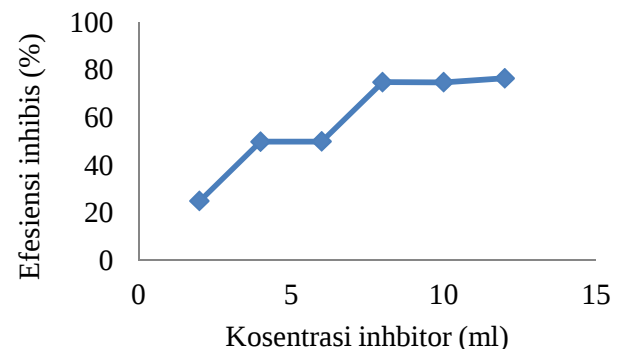
Gambar 2 Hubungan konsentrasi inhibitor terhadap efesiensi inhibis pada medium NaCl 3%.
