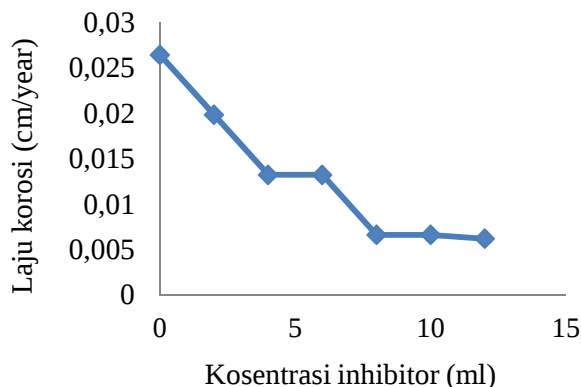
Gambar 1 Pengaruh konsentrasi inhibitor terhadap laju korosi dalam medium NaCl3%.
