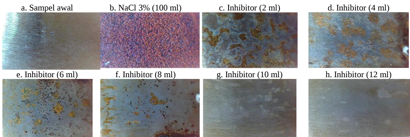
Gambar 3 Foto permukaan sampel setelah perendaman 168 jam dalam medium NaCl 3% dengan dan tanpa penambahan inhibitor
