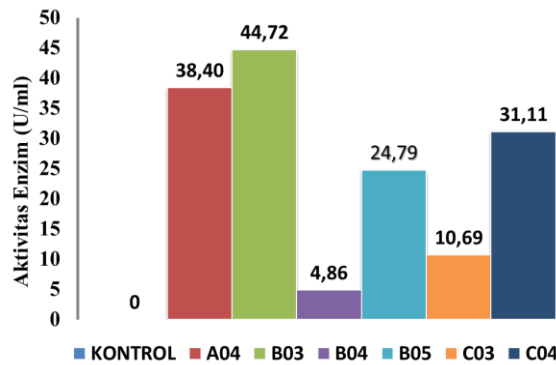
Gambar 6. Grafik aktivitas tinggi enzim tanase dalam reaksi hidrolisis asam tanat oleh 6 isolat bakteri. isolat B03 menunjukkan memiliki aktivitas paling tinggi 44,72 U/ml
