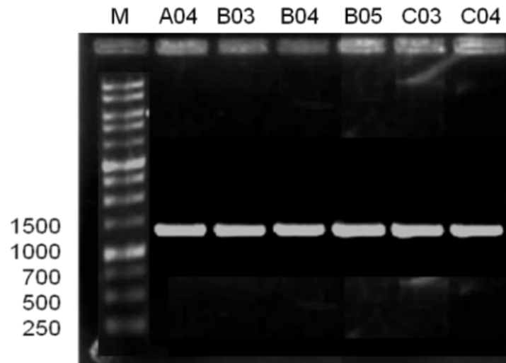
Gambar 7. Elektroforegram produk PCR Gen 16S rRNA 6 isolat bakteri penghasil tanase aktivitas tinggi
