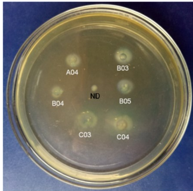
Gambar 5. Zona hidrolisis asam tanat oleh beberapa isolat bakteri
