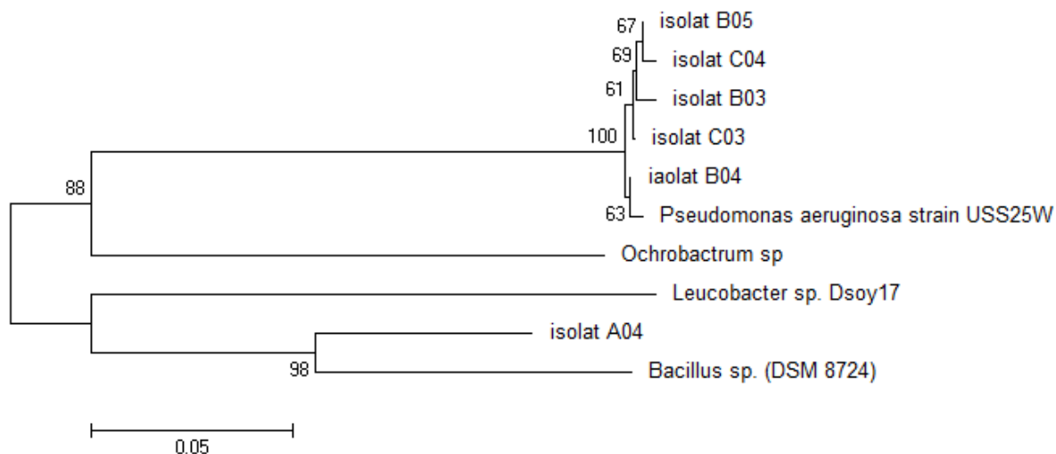
Gambar 8. Pohon filogenetik bakteri penghasil tanase hasil penelitian dengan beberapa bakteri penghasil tanase yang telah ditemukan sebelumnya menggunakan test neighbor-joining tree dengan bootstrap 500 replikasi
