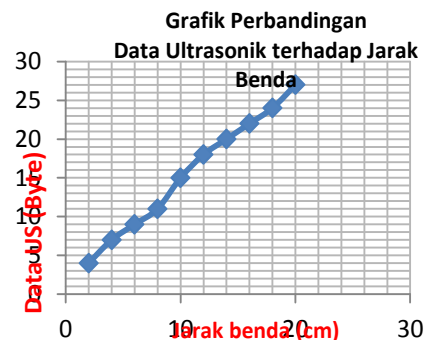
Gambar 19. Grafik Data Ultrasonic Terhadap Jarak Benda
