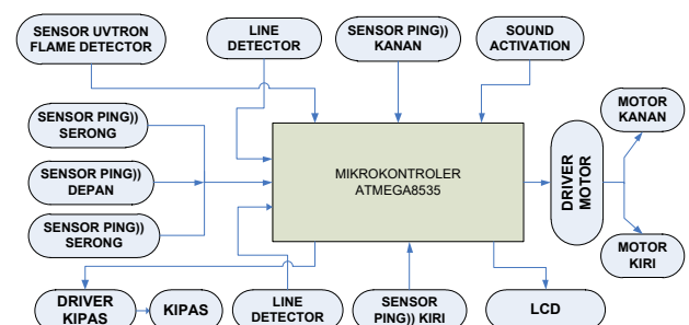
Gambar 5. Blok Diagram Sistem Kendali Robot Pemadam Api
