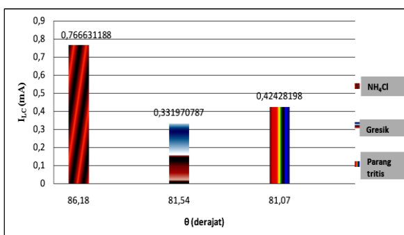
Gambar 8. Grafik sudut kontak ( \theta ) arus bocor rata-rata ( I_{\text{LC}} )
