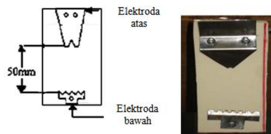
Gambar 2. Penempatan elektroda pada bahan uji.
