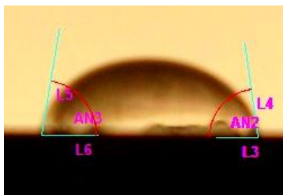
Gambar 6. Pengukuran Sudut kontak resin epoksi dengan kontaminan Pantai Parangtritis
