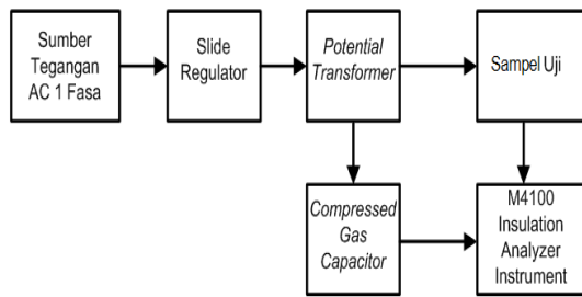
Gambar 7. Diagram blok pengujian \tan \delta
