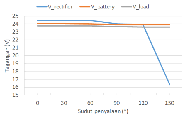
Gambar 10. Tegangan pada sudut penyalan thyristor yang berbeda
