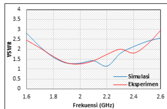
Gambar 7. Grafik perbandingan pengukuran nilai VSWR antena bowtie terintegrasi reflektor AMC hasil simulasi dan eksperimen
