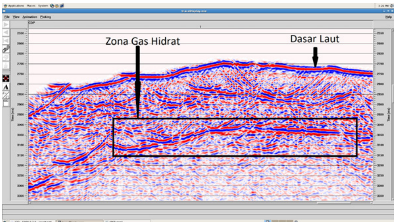
Gambar 9. Kenampakan Bottom Simulating Reflector pada hasil rekaman seismik line 3.01
