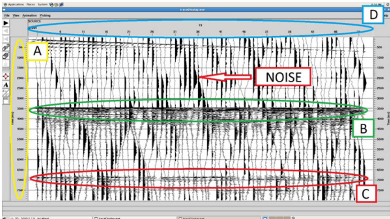
Gambar 6. Hasil rekaman seismik line 3.01: (A) Waktu tempuh; (B) Dasar perairan; (C) Pantulan sekunder/multiple; dan (D) Trace header
