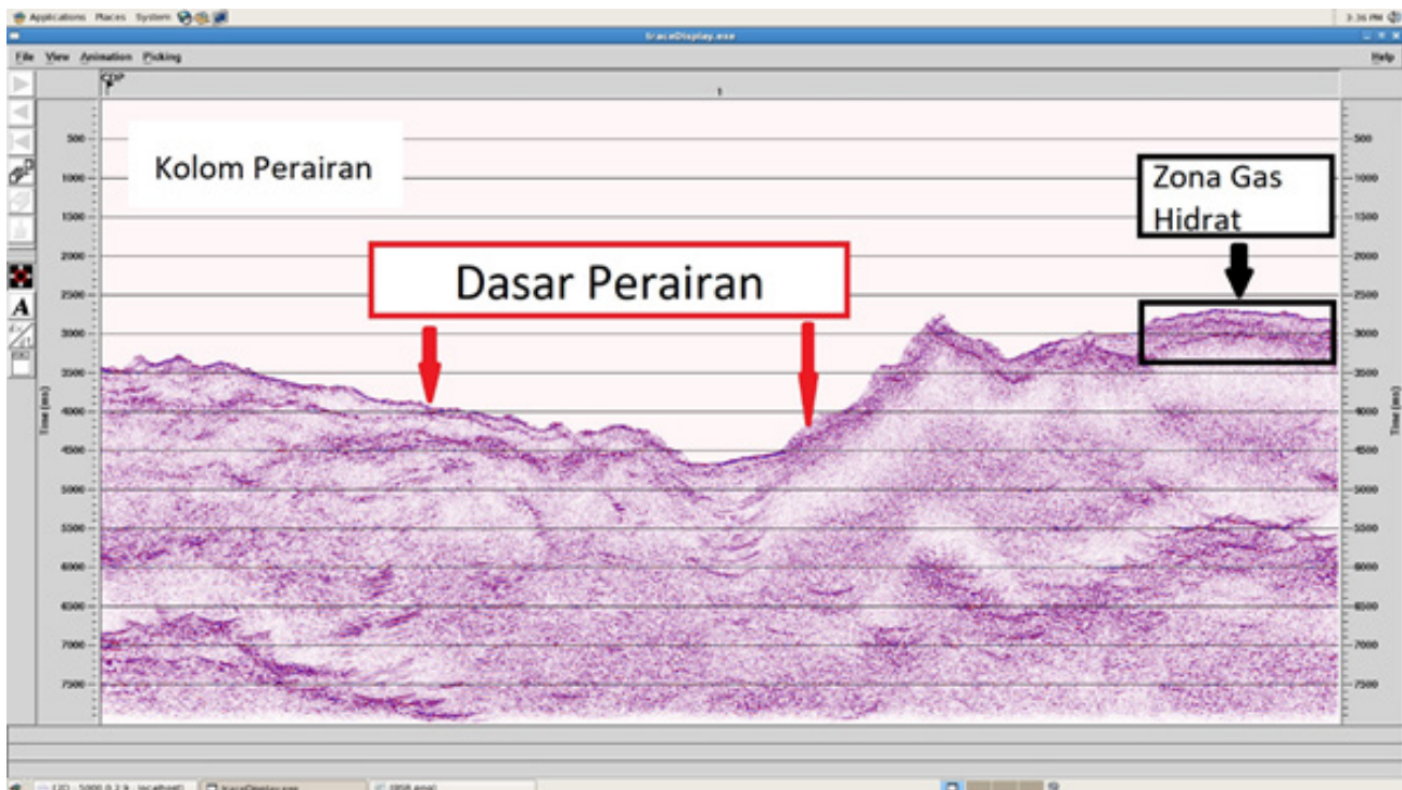
Gambar 8. Hasil rekaman seismik line 3.01 setelah proses stackin dan migrasi
