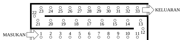
Gambar 5. Posisi pengukur temperatur kolektor dua belokan memanjang 180^\circ
