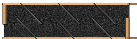
Gambar 3. Tata letak hambatan kolektor dengan lalu multi berbelokan sudut 130^\circ
