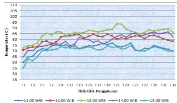
Gambar 8. Distribusi temperatur absorber pada laluan kolektor surya dengan sudut hambatan 130°
