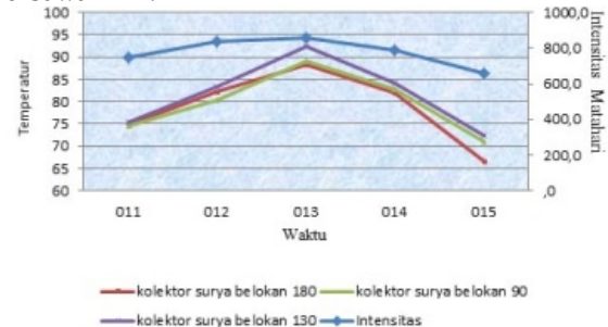
Gambar 11. Titik Tertinggi dari tiga kolektor
