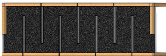
Gambar 1. Tata letak hambatan kolektor dengan lalu berbelokan sudut 90^\circ
