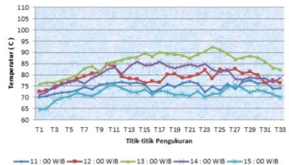
Gambar 7. Distribusi temperatur absorber pada laluan kolektor surya dengan sudut hambatan 90°
