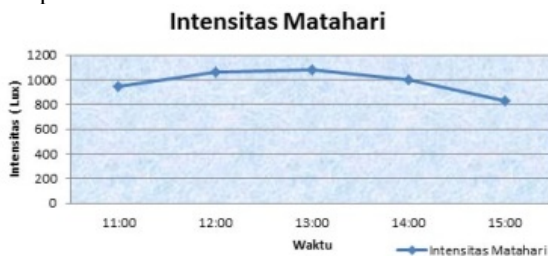
Gambar 10. Distribusi Intensitas Matahari
