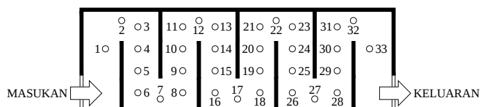
Gambar 2. Posisi pengukur temperatur pada kolektor dengan lalu multi berbelokan sudut 90^\circ
