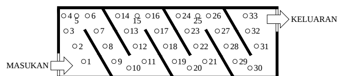
Gambar 4. Posisi pengukur temperatur pada kolektor dengan lalu multi berbelokan sudut 130^\circ
