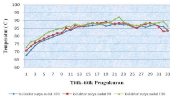
Gambar 9. Grafik Gabungan Antara Ketiga Kolektor
