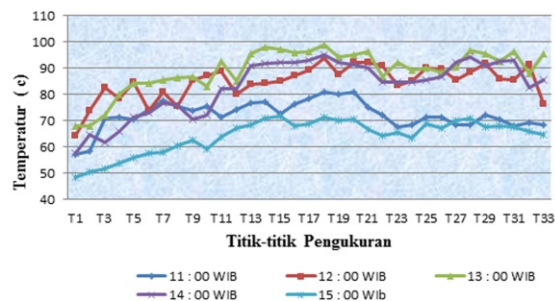
Gambar 6. Distribusi temperatur absorber pada laluan kolektor surya dengan dua belokan memanjang 180°
