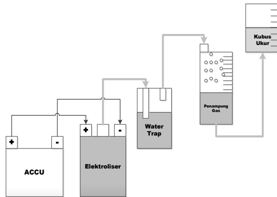
Gambar 2. Skema Pengujian Generator HHO
