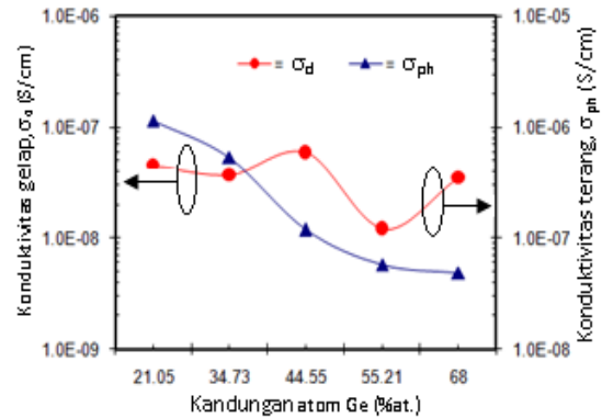
Gambar 4. Pengaruh persentase kandungan Ge terhadap konduktivitas gelap, \sigma_{\text{d}} dan konduktivitas terang, \sigma_{\text{ph}} lapisan tipis a-SiGe:H.
