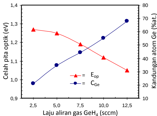
Gambar 3. Pengaruh laju aliran gas \text{GeH}_4 terhadap kandungan atom Ge ( C_{\text{Ge}} ) dan celah pita optik ( E_{\text{opt}} ) lapisan tipis a-SiGe:H.
