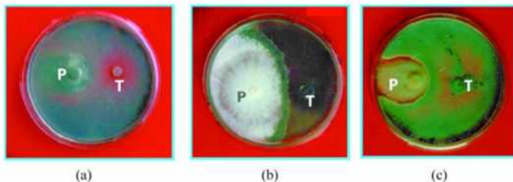
Gambar 7. Tiga mekanisme interaksi antara Trichoderma dan fungi patogen: (a) mikoparasit (b) kompetisi (c) antibiosis, T = Trichoderma P = patogen Ganoderma (Widyastuti 2006)
