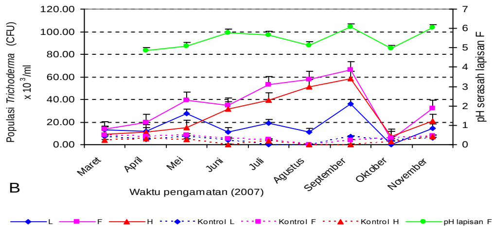
Gambar 3 Fluktuasi populasi Trichoderma dan kondisi pH pada lapisan F serasah A. Mangium Keterangan: A = pada tegakan sehat, B = pada tegakan terserang Ganoderma , bar = standard error
