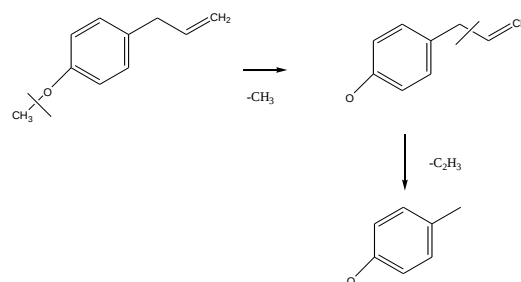
Gambar 1. Pola Pragmentasi Estragol
